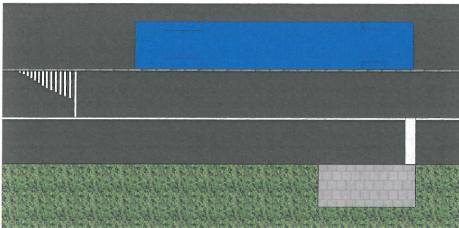
Principskiss: Cykelfält förbi hållplats utan ficka
