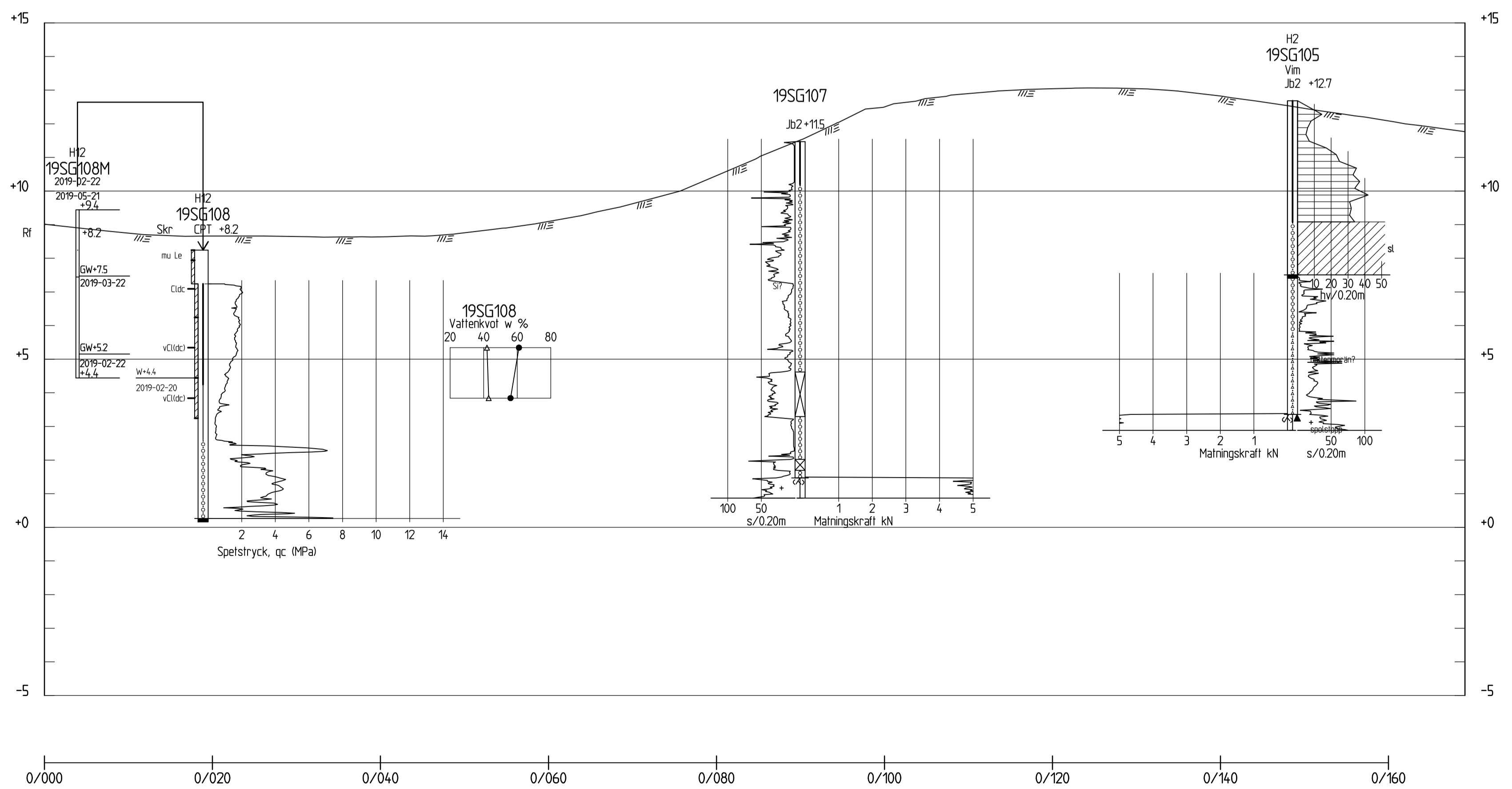
SEKTION B-B H 1:100 L 1:400
