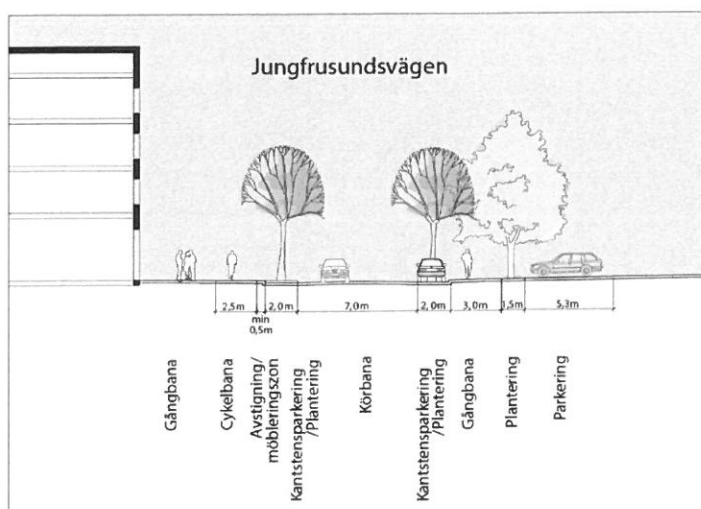
Gatusektion genom Jungfrusundsvägen i sydost
