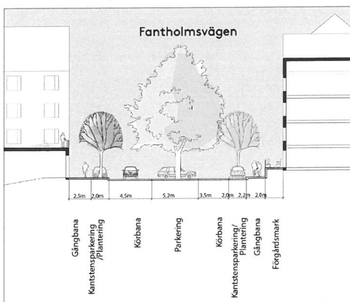
Gatusektion genom Fantholmsvägen
