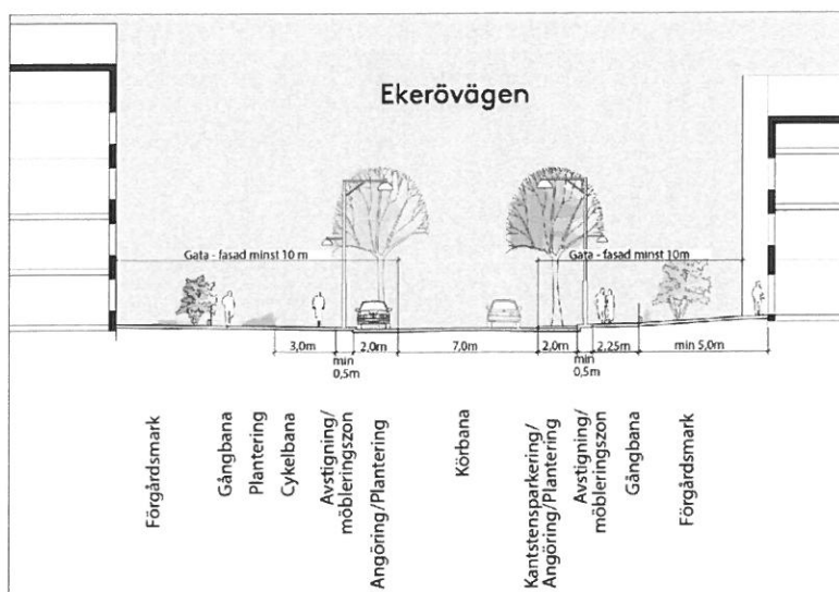
Gatusektion genom Ekerövägen vid bostadsbebyggelsen i nordost
