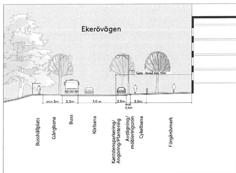
Gatusektion genom Ekerövägen vid bostadsbebyggelsen i sydväst
