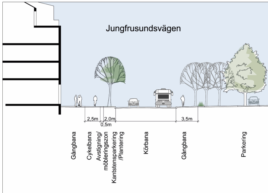
Gatusektion/typsektion genom Jungfrusundsvägen i riktning mot nya Träkvista torg från sydost
