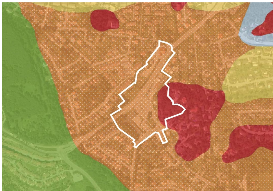
Utdrag från Geoteknisk sektorsportal (hämtat 2018-04-10); orange – postglacial sand, grönt – isälvsediment, rött – urberg, gul – postglacial lera, blå – sandig morän
