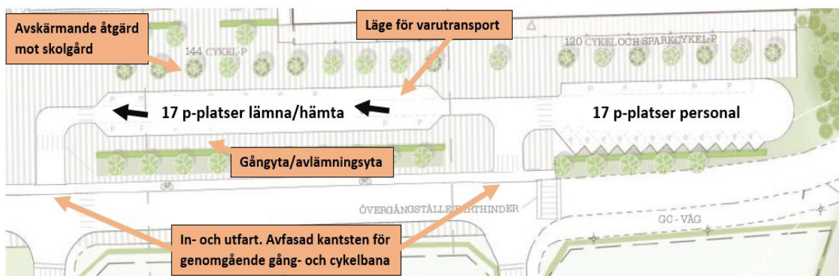
Figur 15, förslag på utformning av angöringsgata
