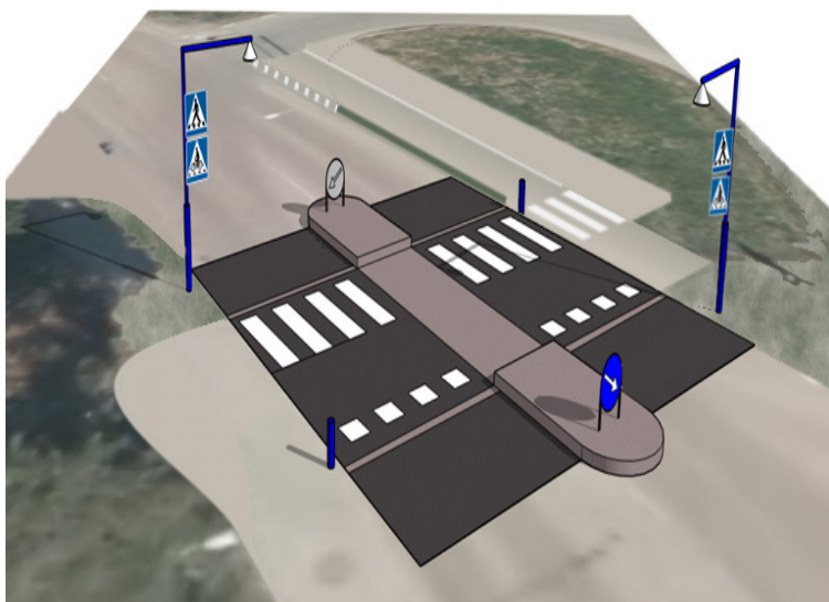
Figur 19, förslag på utformning av övergångsställe med belysning
