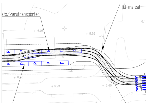
Figur 24, förslag på in och utfart för varustransporter i slingan. Lastbilen angör i slingan. Dessa platser bör skyltas som lastplats under angiven tid. Parkeringsplatser på slingans norra sida bör göras 2,5 meter breda i detta fall. Körspår med LBN (tung lastbil).
