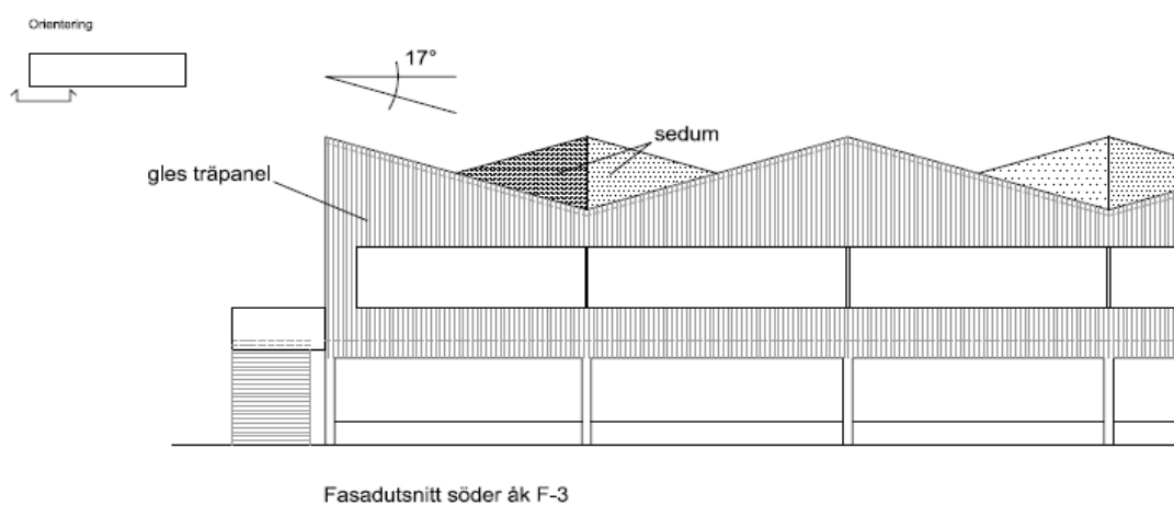
Figur 12, fasadutsnitt för utformning av tak med upprepande sadeltaksmotiv
