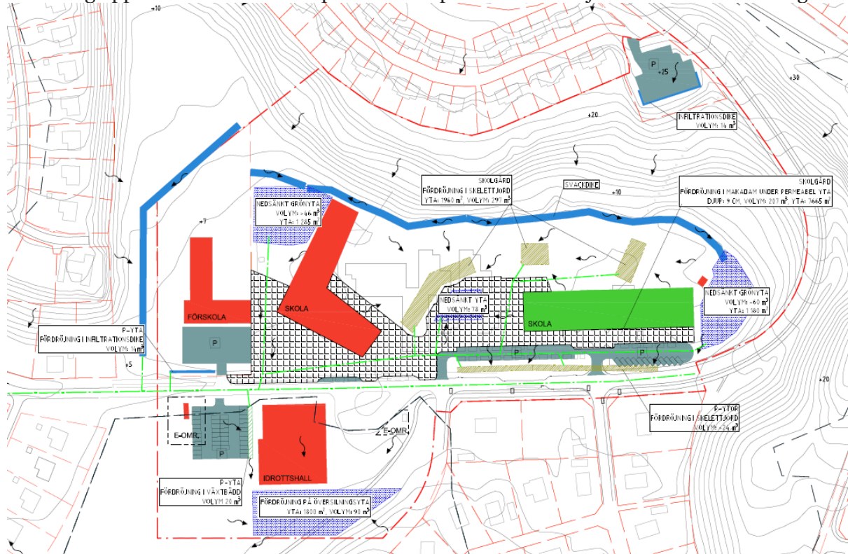
Figur 26, skiss över föreslagen dagvattenhantering från fördjupad dagvattenutredning (ÅF-Infrastructure AB, 2019-10-21)
