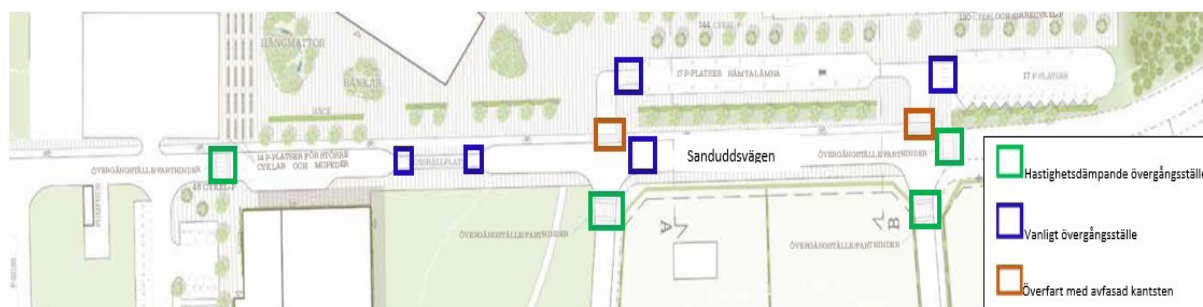
Figur 18, förslag på placering av övergångsställen
