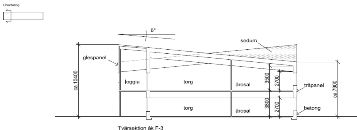
Figur 11, tvärsektion för utformning av tak med upprepande sadeltaksmotiv
