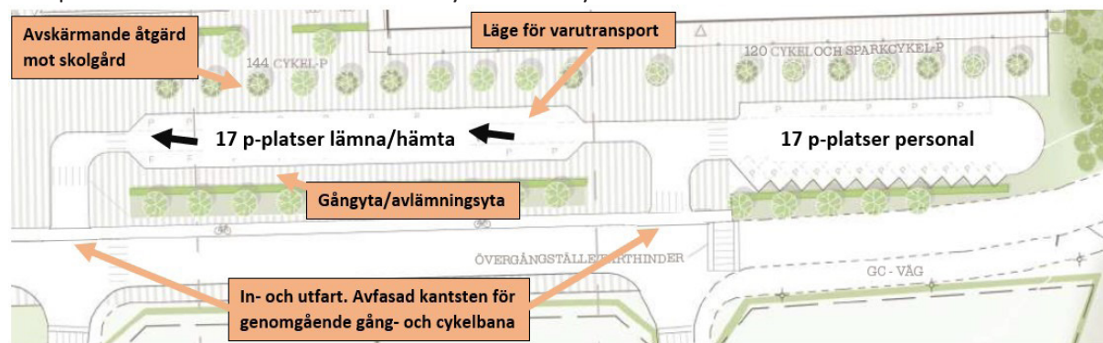
Figur 23, förslag på utformning av angöringsslinga samt parkering
