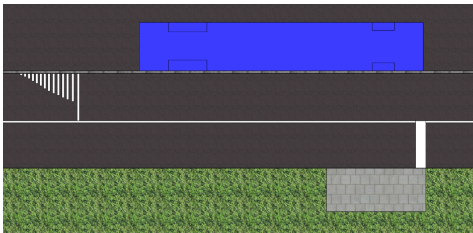
Principskiss: Cykelfält förbi hållplats utan ficka
