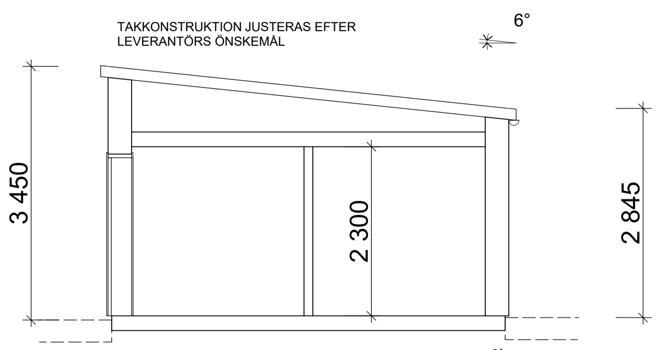
A-A TVÄRSEKTION
