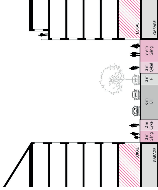
Gatusnitt Ångbåtsvägen 1:400
