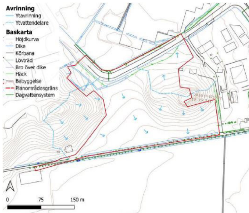
Fig 30. Befintlig dagvattenhantering och ytlig avrinning i området (WRS)
