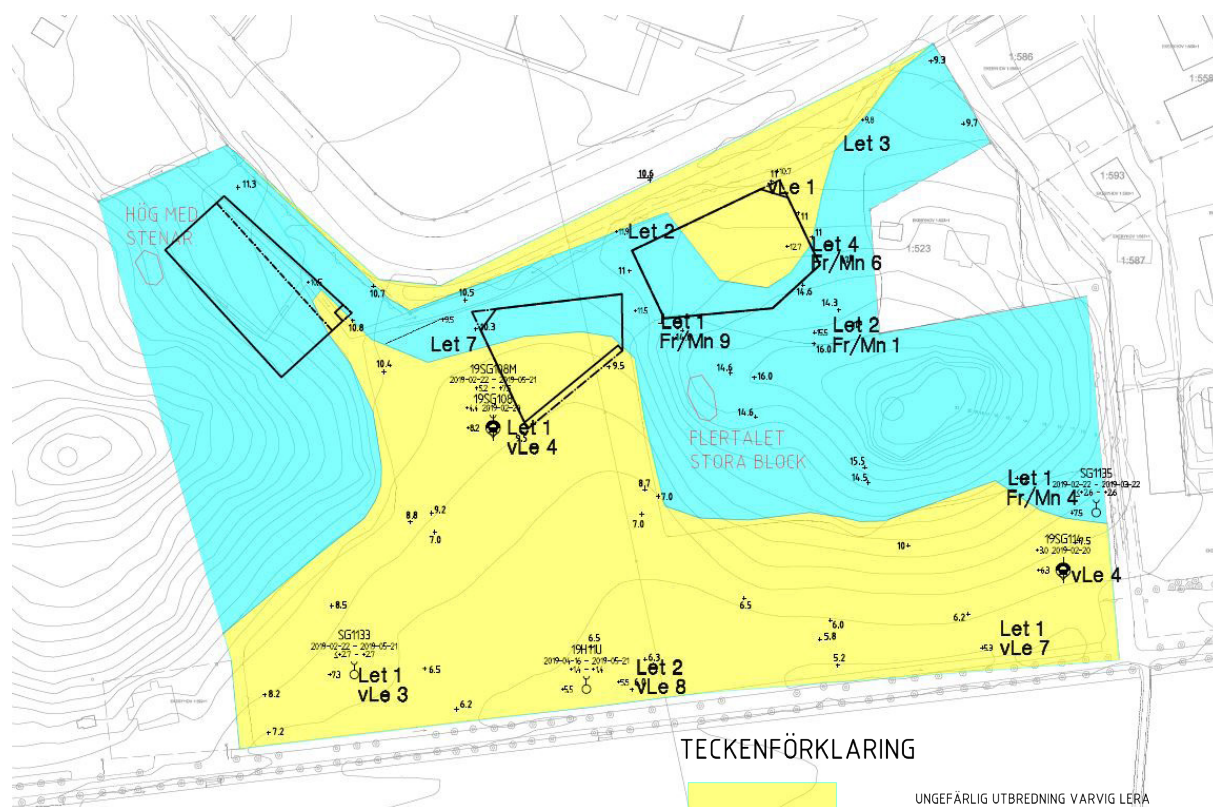
Fig 10. Markförhållanden i området (Structor).
