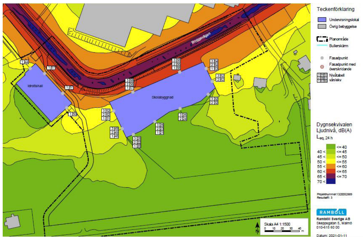
Fig 35. Ekvivalenta bullernivåer år 2040 (Ramböll, 2021-01-29, rev. 2021-09-02)
