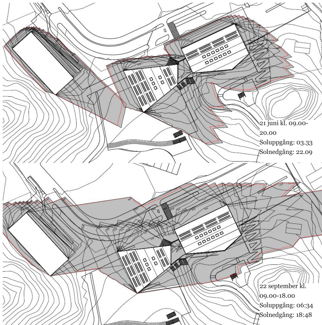
Fig 40-41. Skuggpåverkan av skolbyggnad, redovisad per timme (LLP Arkitektkontor). Grå skuggning visar högsta tillåtna nockhöjd och röd linje visar föreslagen skolbyggnad.
