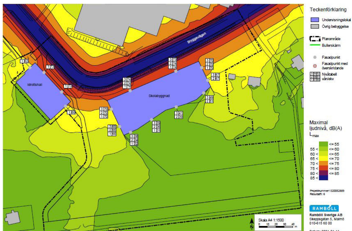
Fig 36. Maximala bullernivåer år 2040 (Ramböll, 2021-01-29, rev. 2021-09-02)
