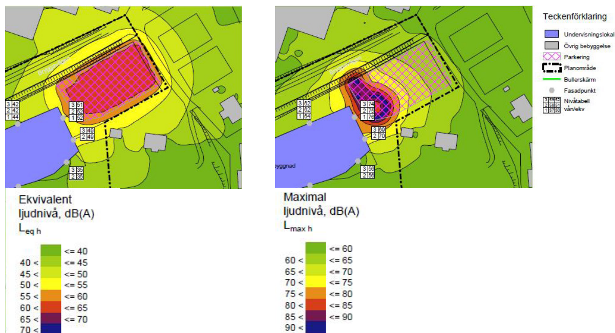
Fig 37. Ekvivalenta respektive maximala bullernivåer från personalparkering (inkl. transporter). (Ramböll, 2021-01-29, rev. 2021-09-02)
