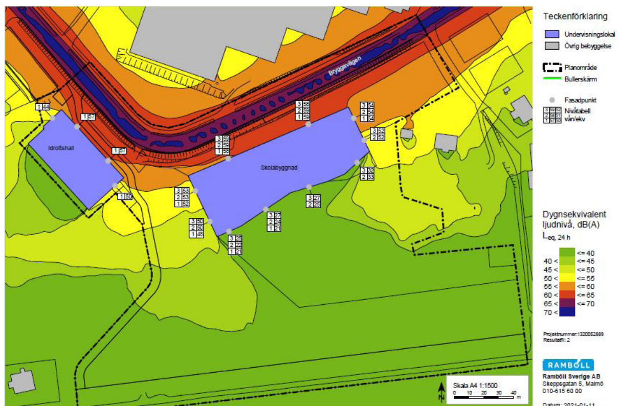
Fig 33. Ekvivalenta bullernivåer år 2020 (Ramböll, 2021-01-29, rev. 2021-09-02)
