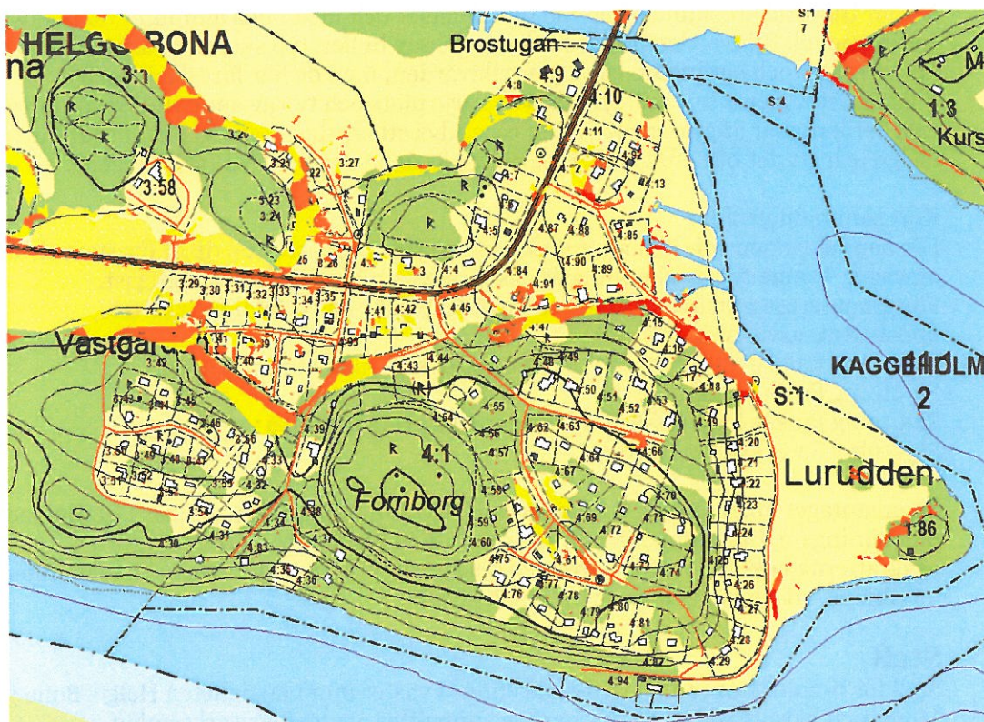
Utdrag ur övergripande ras- och skredriskanalys.
