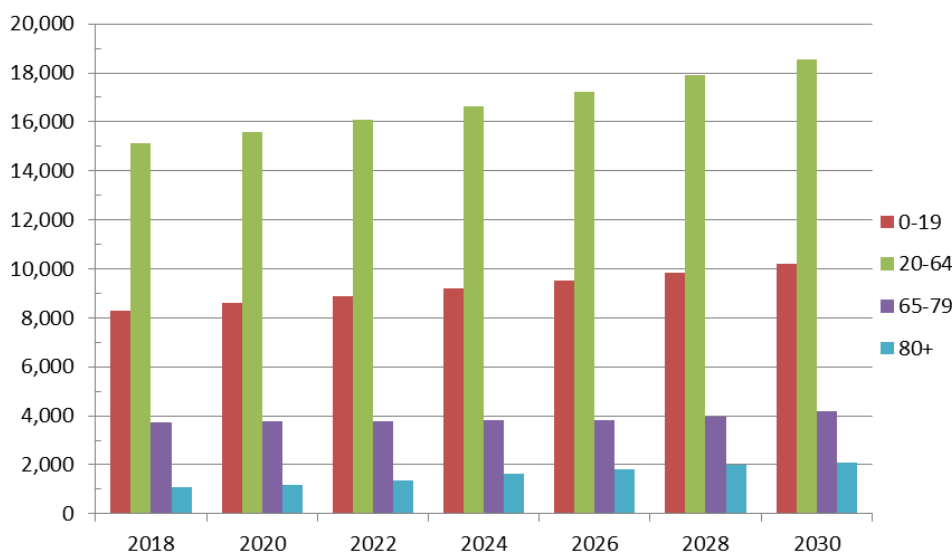
Diagram 1: Befolkningsprognos 2018-2030
