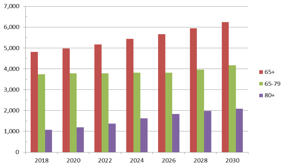
Diagram 2: Befolkningsprognos 65+ 2018-2030
